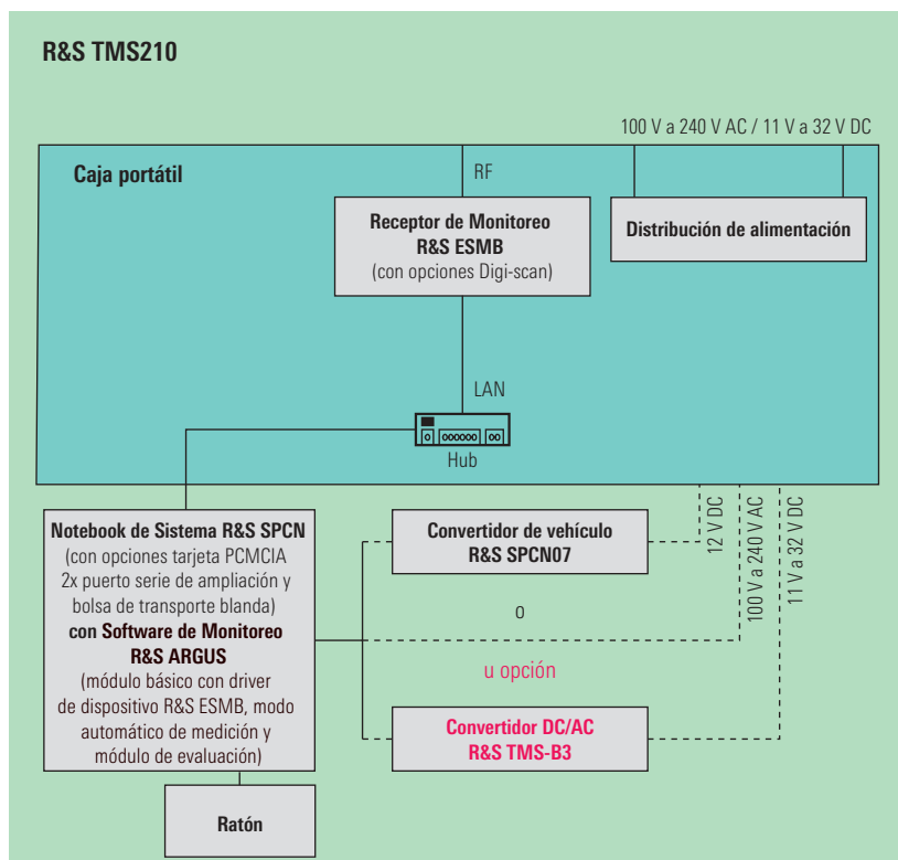
Esquema funcional de R&S TMS210
