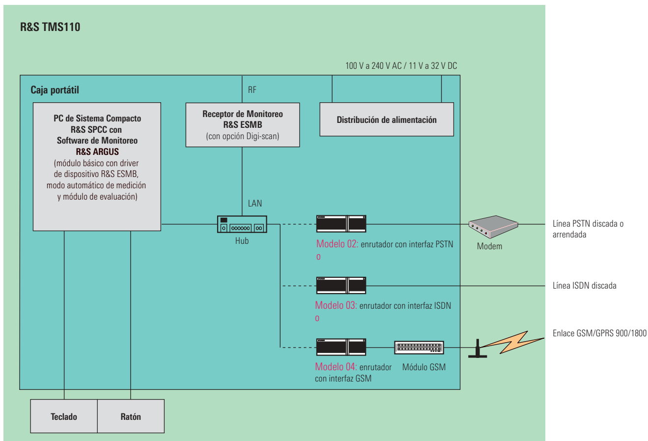
Esquema funcional de R&S TMS110
