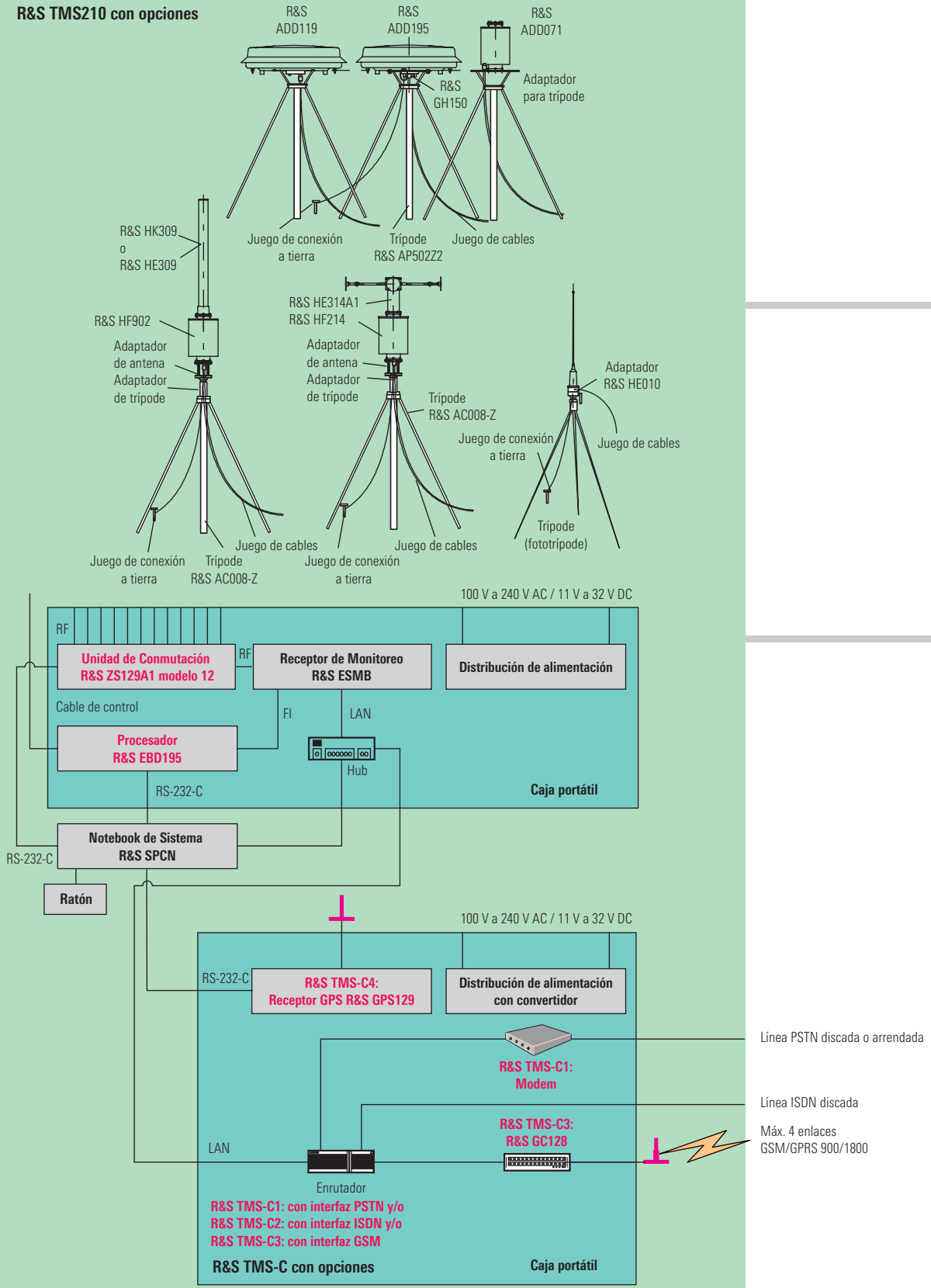
Ejemplo de un R&S TMS 210 con opciones
