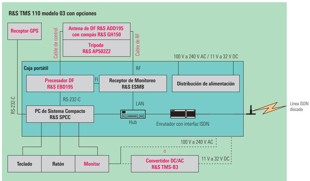
Ejemplo de un R&S TMS 110 modelo 03 con opciones
